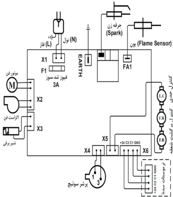
نقشه برق سیستم کنترلی سدنا
