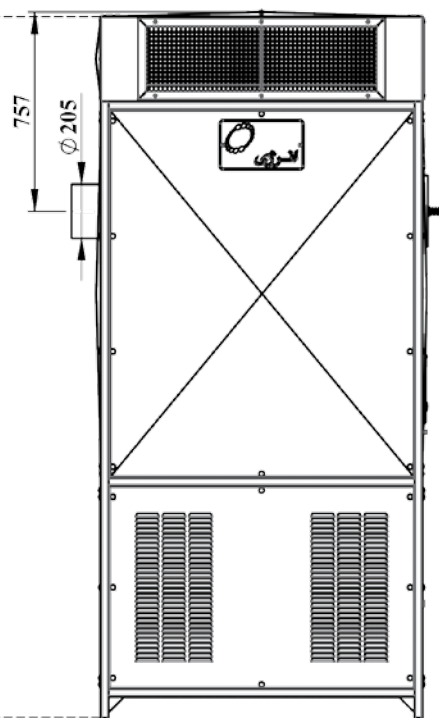
نمای جانبی
