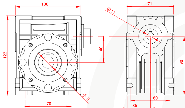
فریم 63
