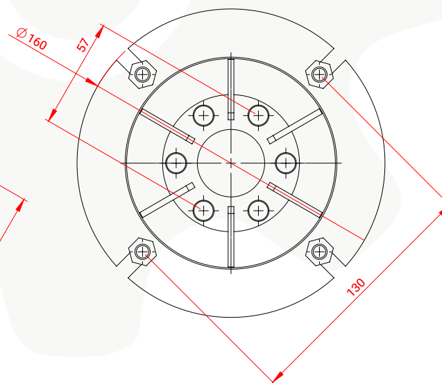
71B14
