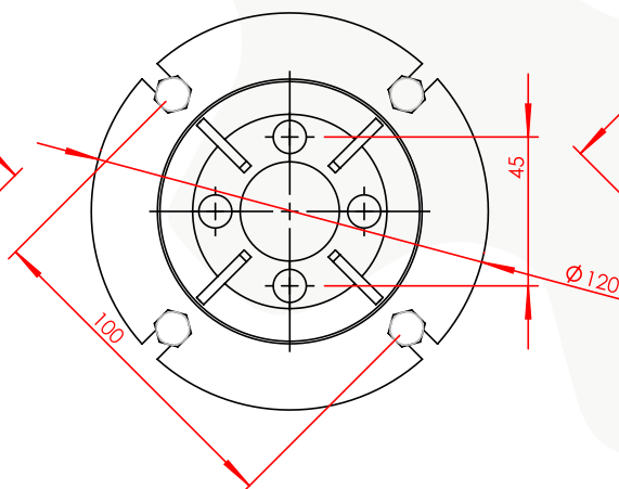
56B5
