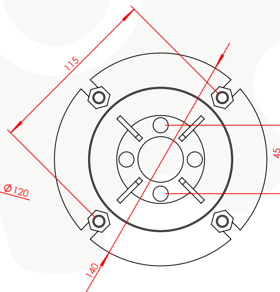
63B5
