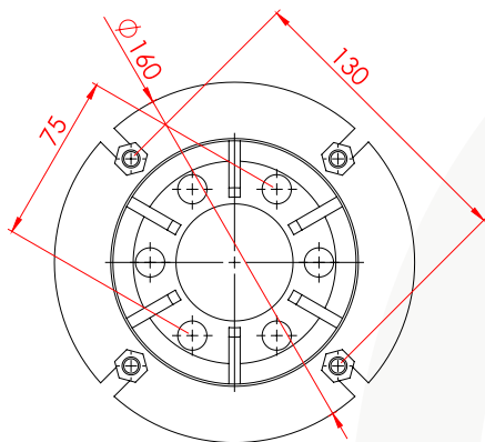
71B5
