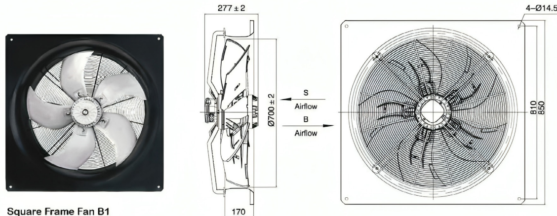
Square Frame Fan B1
