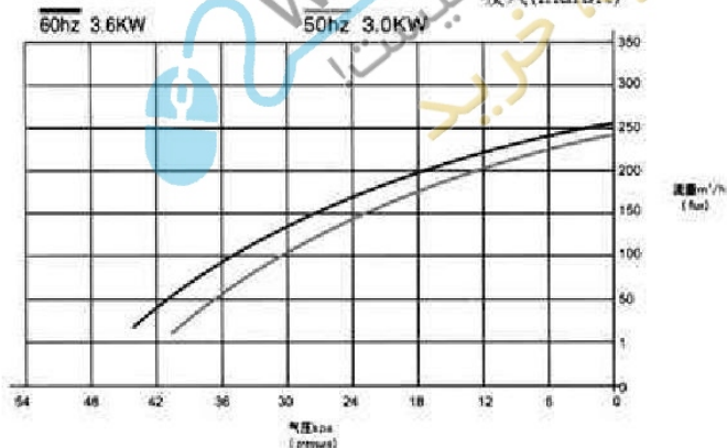
HG系列旋涡气泵性能曲线 (仅供参考不作检测依据)
